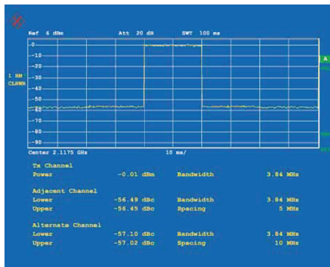
Измерение мощности соседнего канала во временной области
