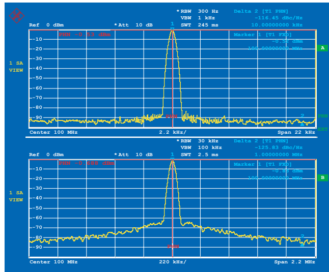
Измерение фазового шума с помощью R&S® FSP
