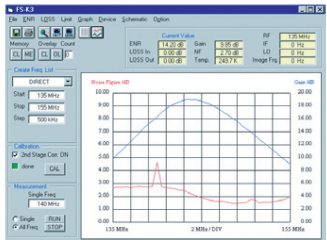
Определение коэффициента шума с помощью программного обеспечения R&S®FS-K30.
