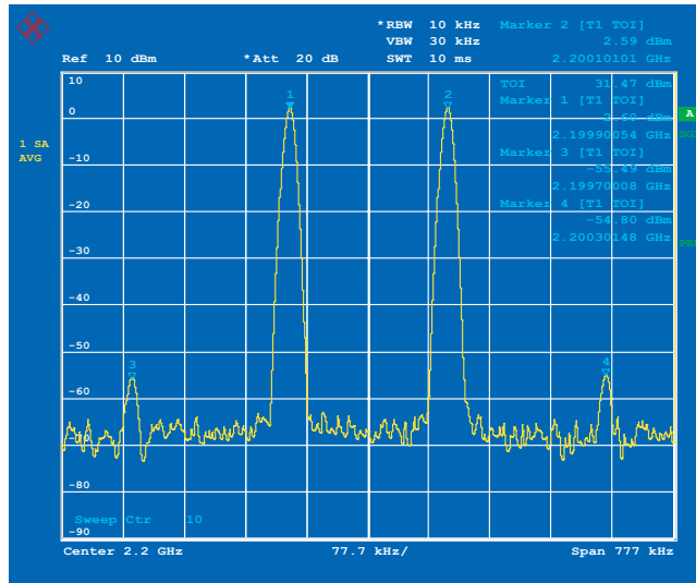
Измерение интермодуляционных искажений 3-го порядка
