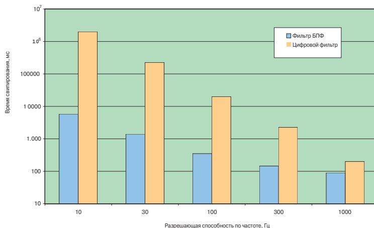
Сравнение времени свипирования для полосы обзора 200 кГц с использованием цифровых фильтров и фильтров БПФ
