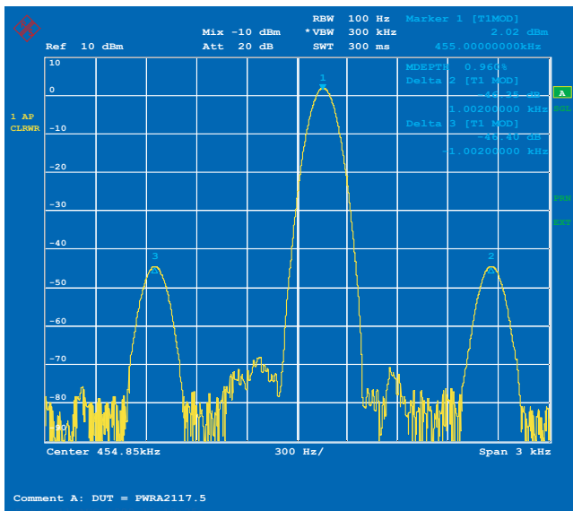
Измерение глубины модуляции AM сигнала
