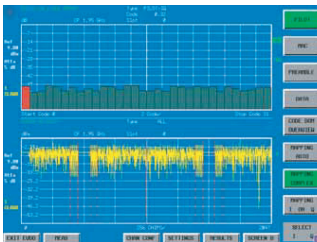
Мощность ошибки и мощность слота для 1xEV-DO сигнала, измеренные при помощи R&S®FS-K84
