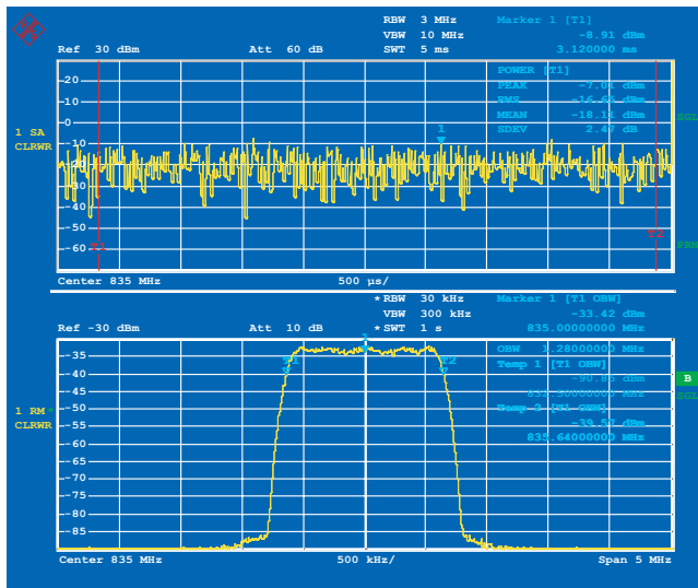
Измерение мощности пакета (верхний график) Определение занимаемой полосы частот (нижний график)
