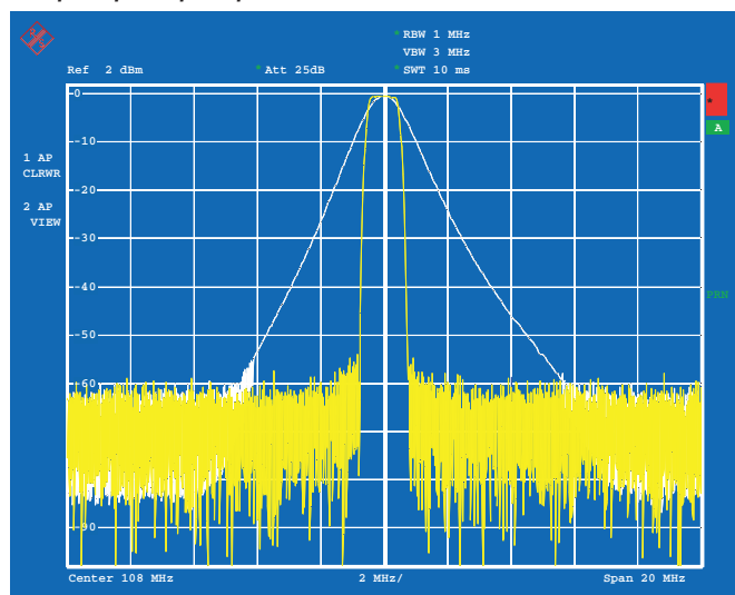
Сравнение канального фильтра на 1 МГц и обычного фильтра с полосой 1 МГц
