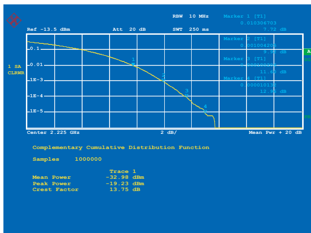
Измерение комплементарной функции распределения WCDMA сигнала
