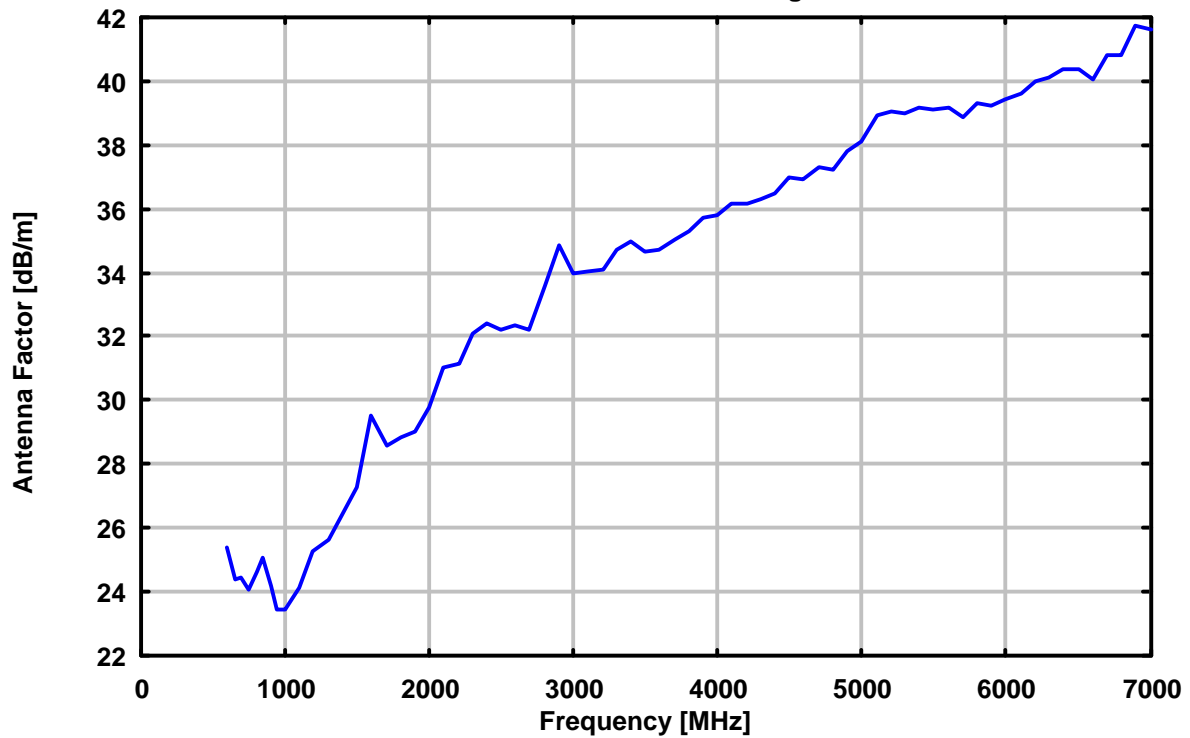
USLP 9142 Antennen-Wandlungsmass
