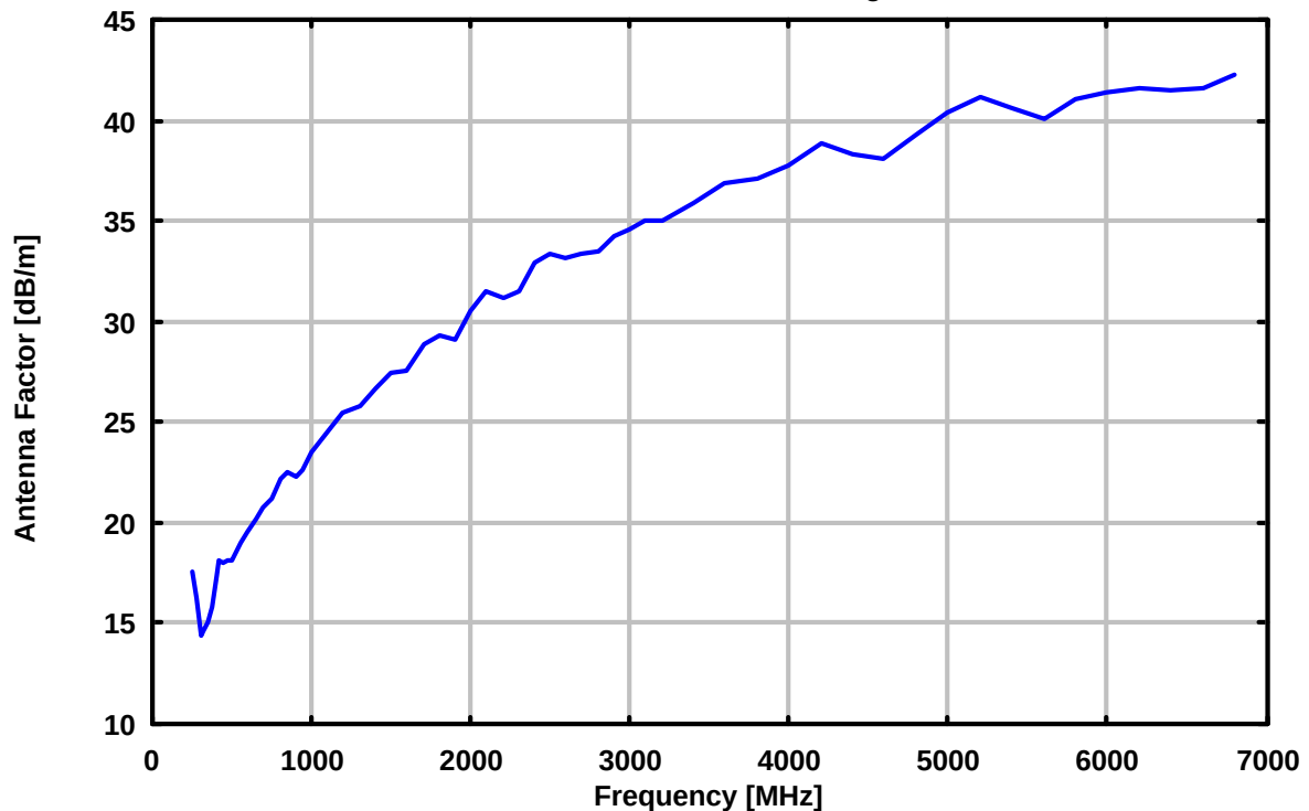
USLP 9143 Antennen-Wandlungsmass
